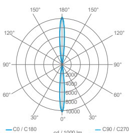
Optic 2x11°
