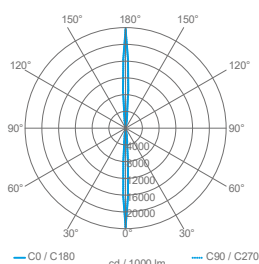
Optic 2x11°
