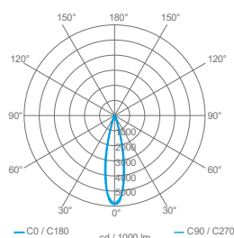
Optic 23°
