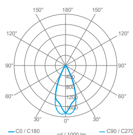
Optic 43°
