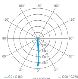
Optic 11°
