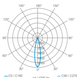
Optic 22°
