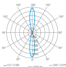
Optic 2x22°
