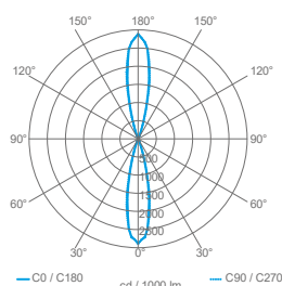
Optic 2x23°
