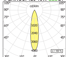
IFERROSI 120 18W LED21°
