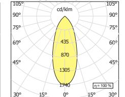
IFERROSI 120 18W LED39°
