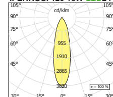
IFERROSI 120 18W LED24°
