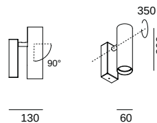
IFERROSI 60 6,7W LED38°
