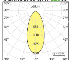
IFERROSI 60 6,7W LED38°
