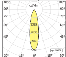
IFERROSI 60 6,7W LED24°
