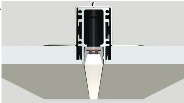
installazione in cartongesso installation in plasterboard
