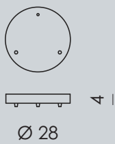
CIELINO TONDO 3 LAMPADE ROUND CEILING 3 LAMPS SU.G3
