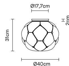
SOFFITTO Ø40 cm / CEILING LAMP Ø40 cm
